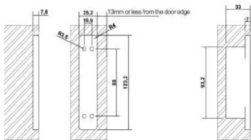
Door frame
